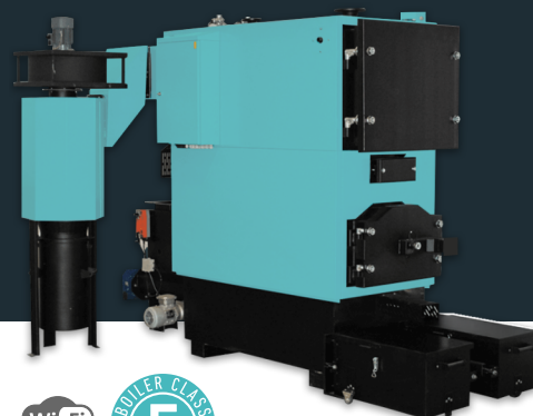
EKO CKS Multi Plus
