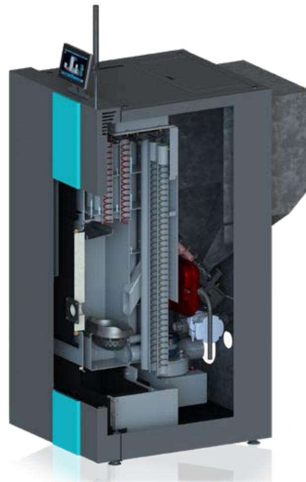
Presjek kotla
