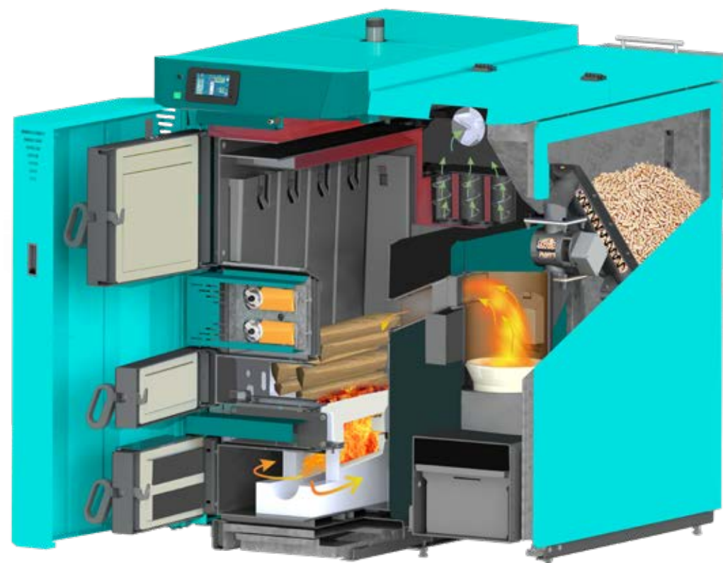
Presjek kotla
