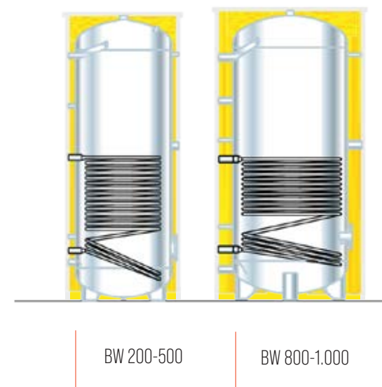
Presjek BW
