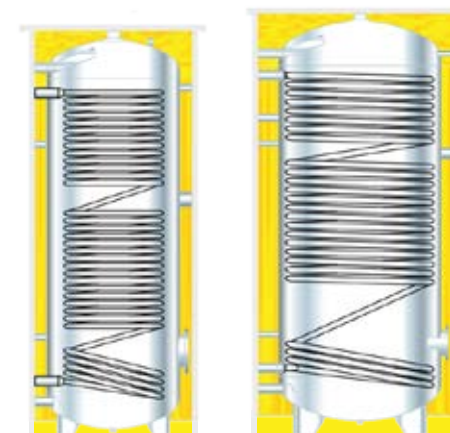
Presjek WWM
